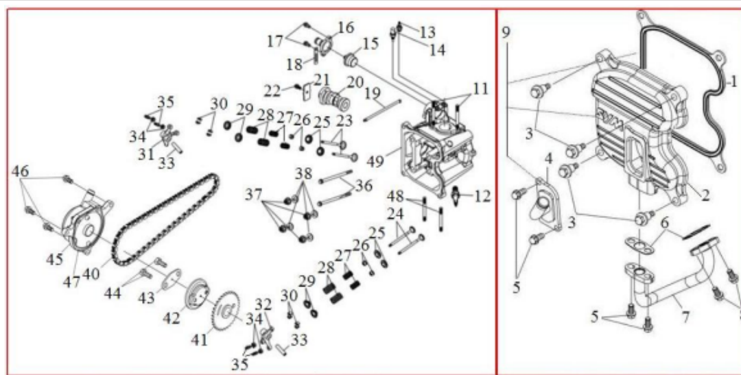
CABEÇOTE / COMANDO DE VÁLVULAS
