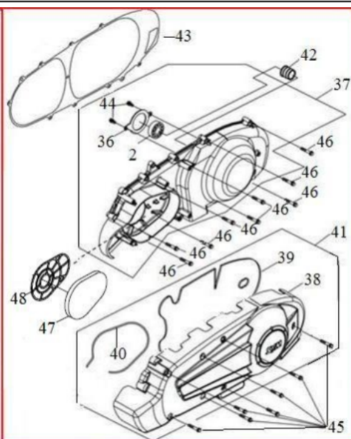
TAMPA LATERAL LE
